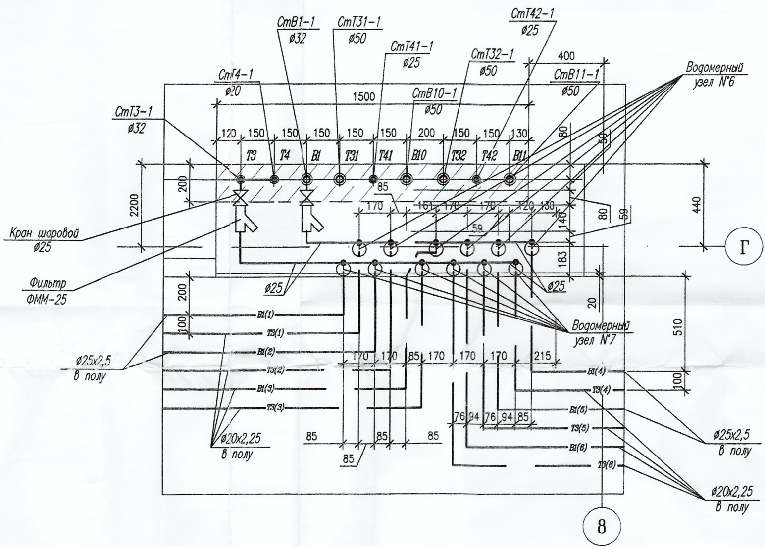
2 зона (4-14 этажи)
